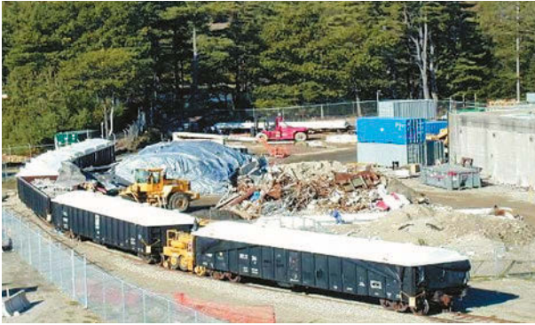
Рис. 3. Погрузка отходов при выводе из эксплуатации АЭС Maine Yankee [17]
