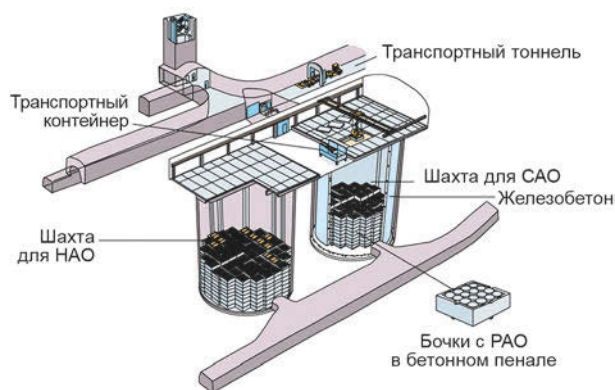
Рис. 5. Проект подземного ПЗРО VLO Olkiluoto repository [16]
